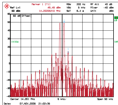
Bild 6: Intermodulation bei 14 MHz im Halb-Modus mit 400 W PEP
