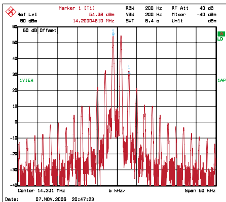
Bild 11: Intermodulation bei 14 MHz und mit voller Leistung
