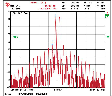
Bild 10: Intermodulation bei 14 MHz und mit 800 W PEP
