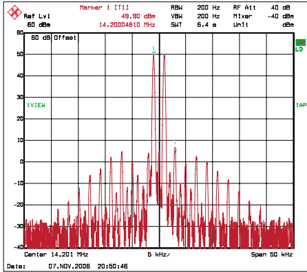
Bild 8: Intermodulation bei 14 MHz und mit 400 W PEP
