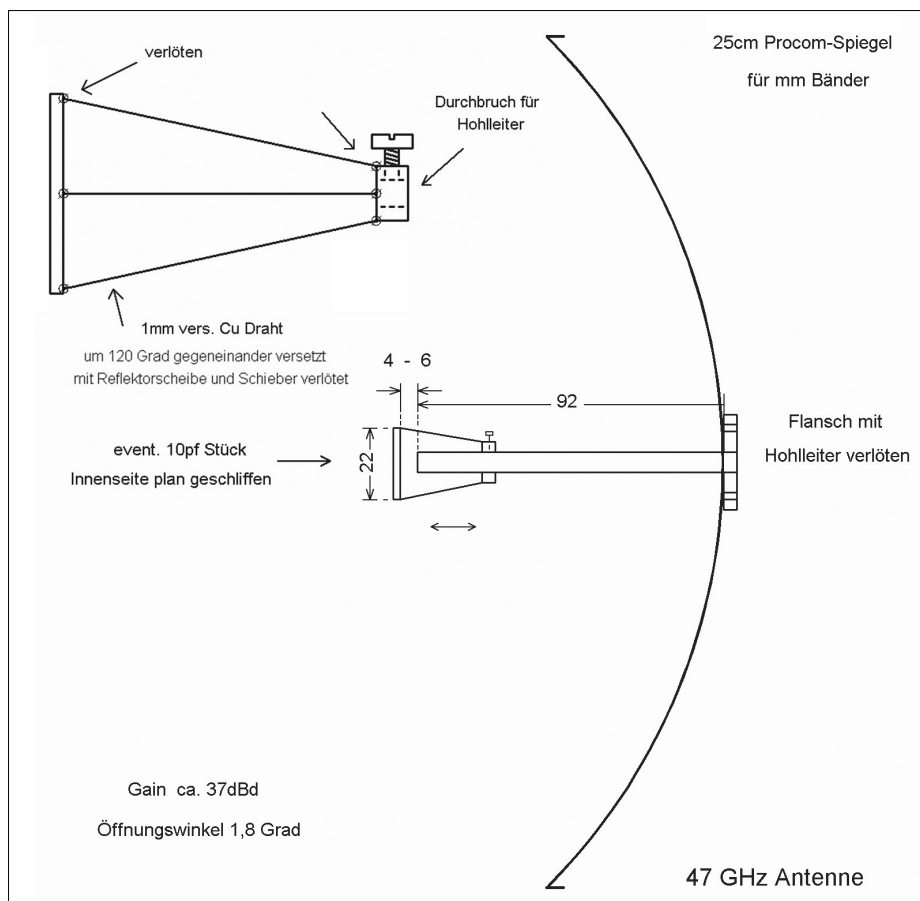
Anhang 2: Zeichnung Spiegel
